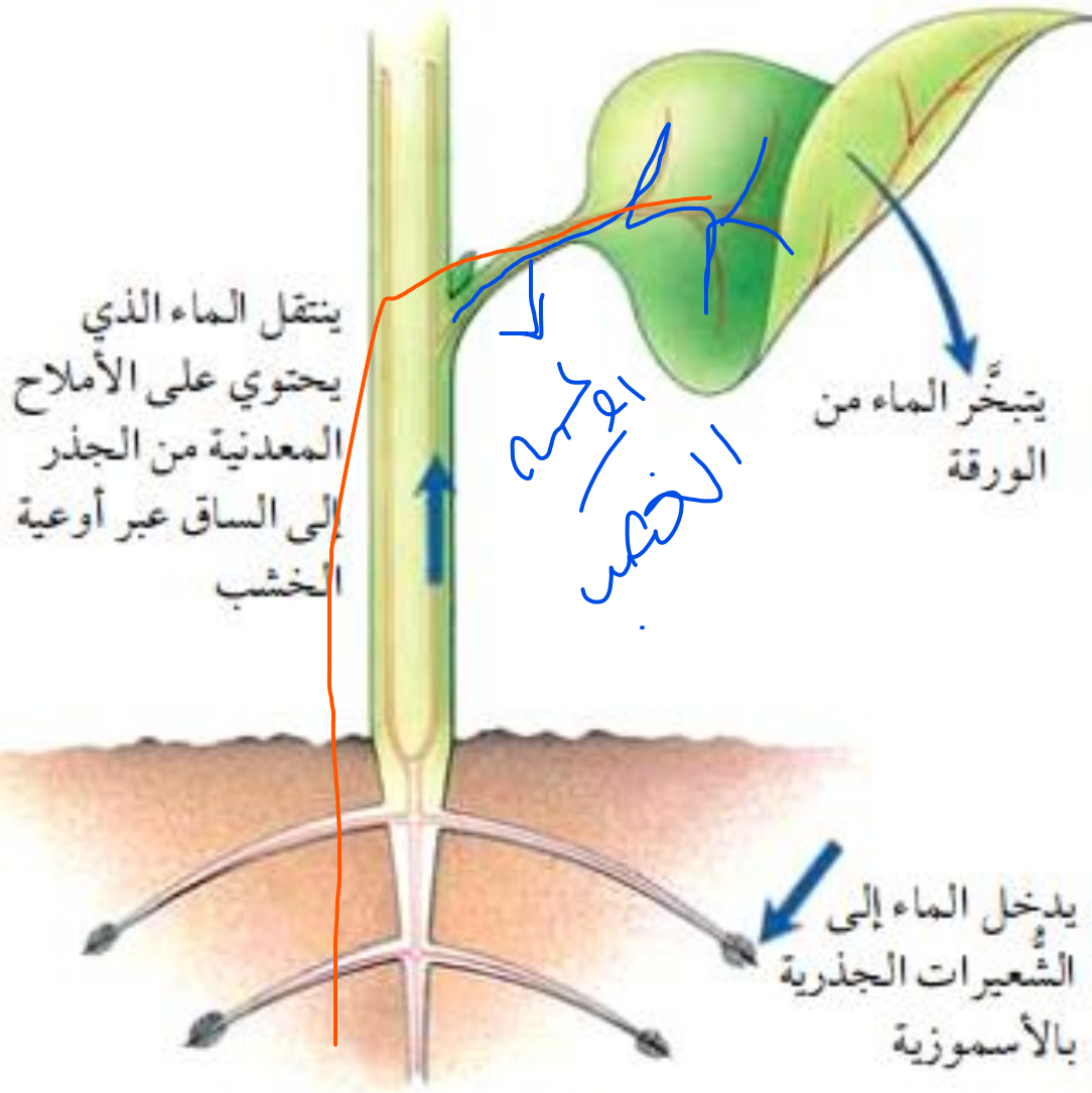
الشكل ٩-٦ تيار النتح
